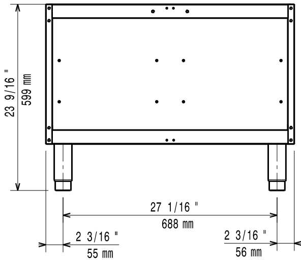
Oldalnézet
